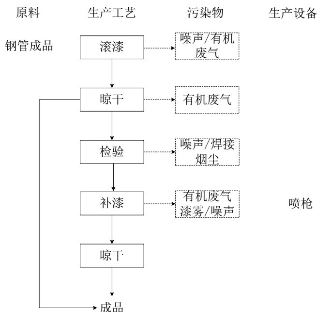
图 2-2 项目滚漆生产工艺流程及产污环节示意图
