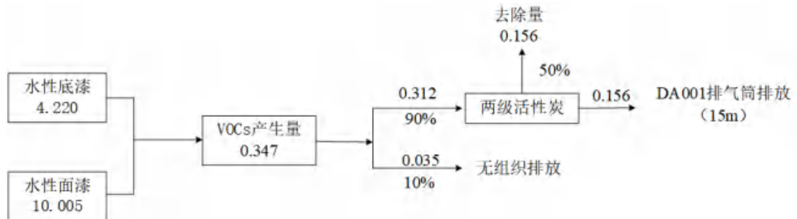
图2-1 项目扩建后VOCs平衡图（单位：t/a）
