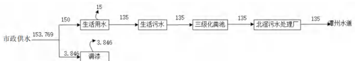
图2-2 项目扩建后水平衡图（单位：t/a）
